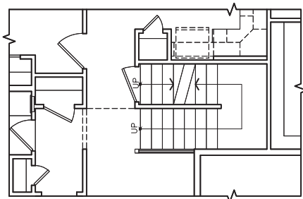
OPT. BAS. / LOFT STAIR PLAN
